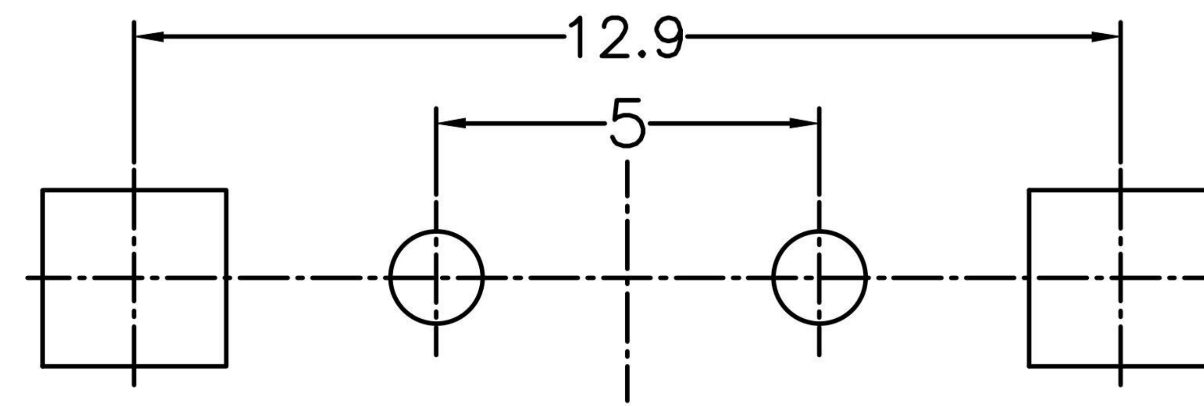
P.C.B LAYOUT
